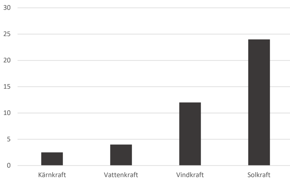
Figur 25 – Livscykelutsläpp för fossilfria energislag, CO 2 g/kWh.
