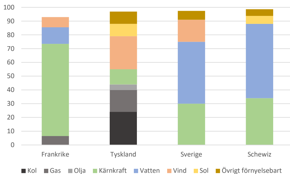
Figur 24 – Jämförelse av elproduktion, 2020.
