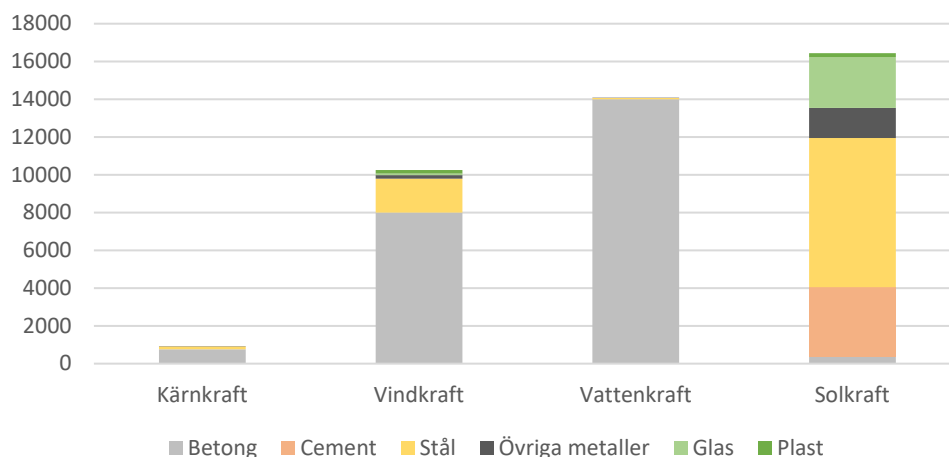
Figur 26 – Resursåtgång för olika energislag, ton per TWh.
